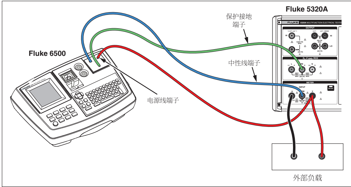
图7-22.使用单独电线进行的电压和电流表校准
