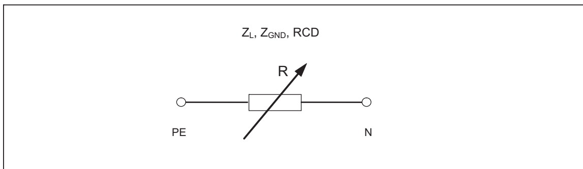
图4-5.简化的接地连接电阻源
