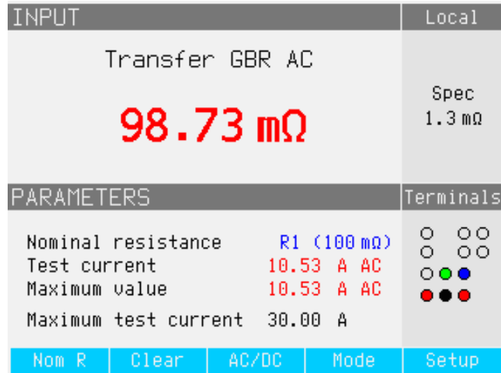
图4-8.传递接地连接电阻显示
