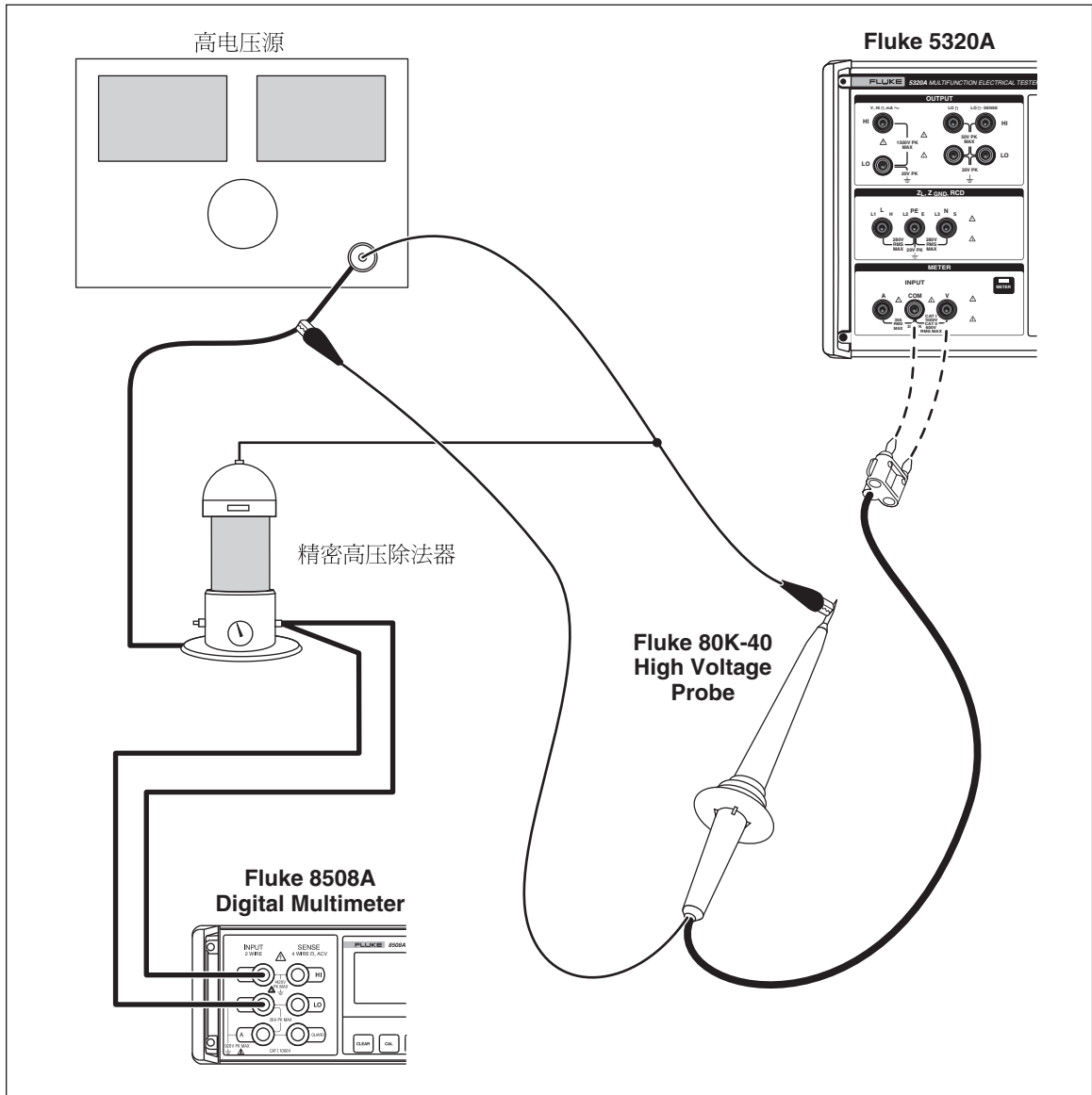
图6-11.高压除法器校准连接
