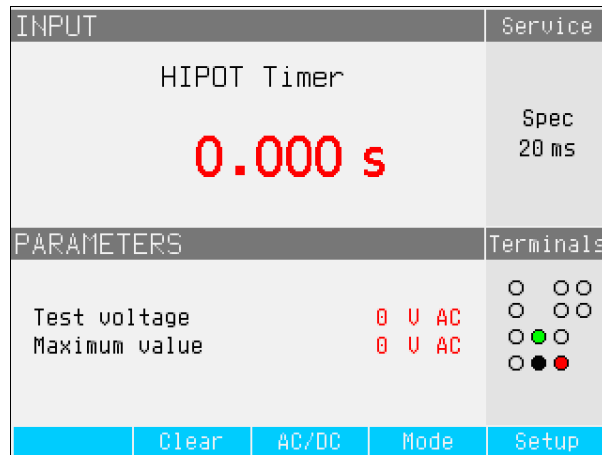
图4-25.有高电位计时器测量值的万用表显示
