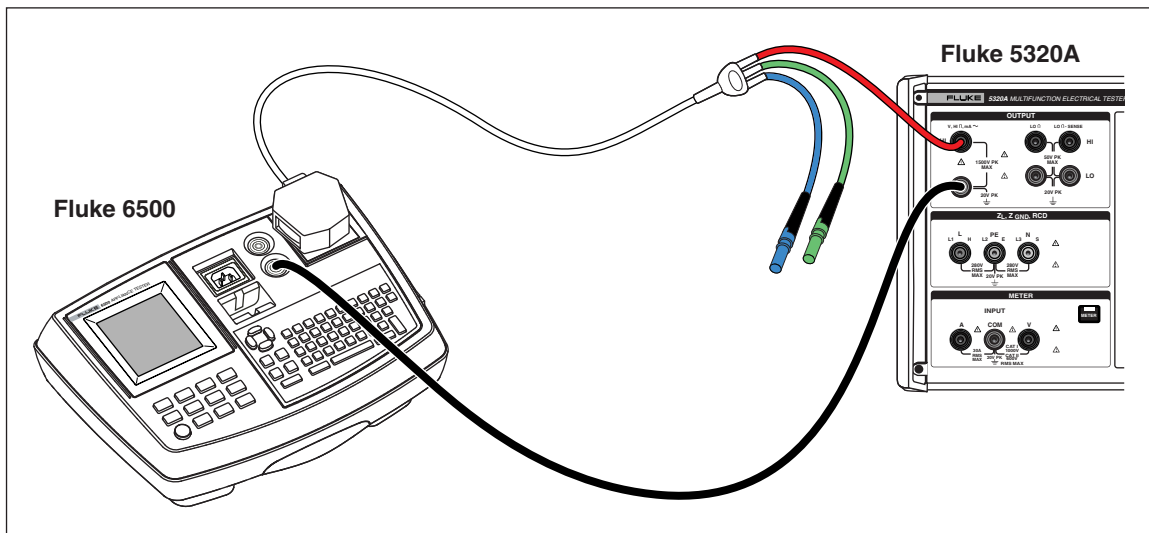
图7-5.校准便携式电器测试仪的绝缘电阻
