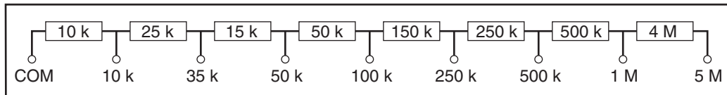
图7-25.负载示意图
