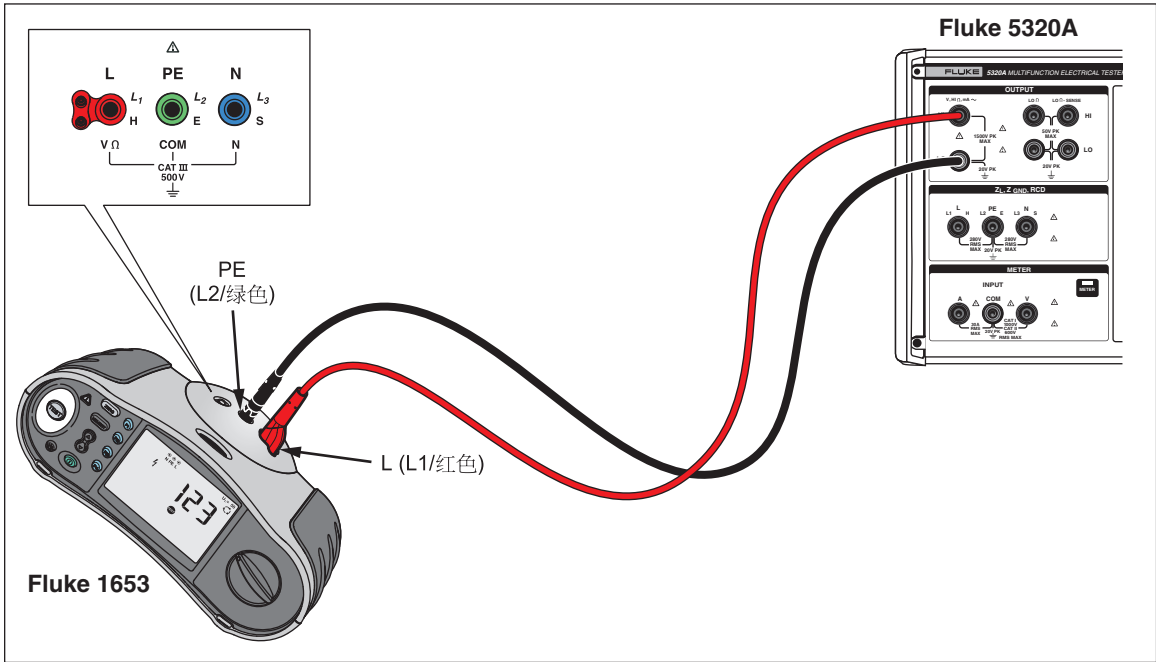
图7-3.校准装置测试仪的绝缘电阻
