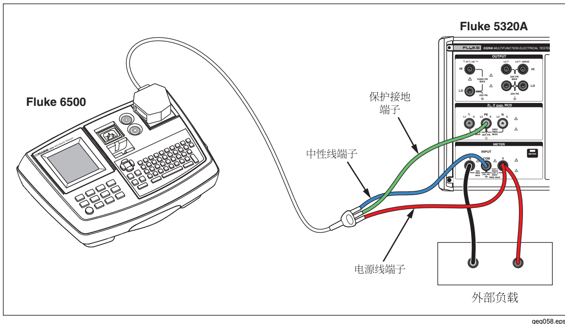
图7-21.使用电缆适配器进行的电压和电流校准。
