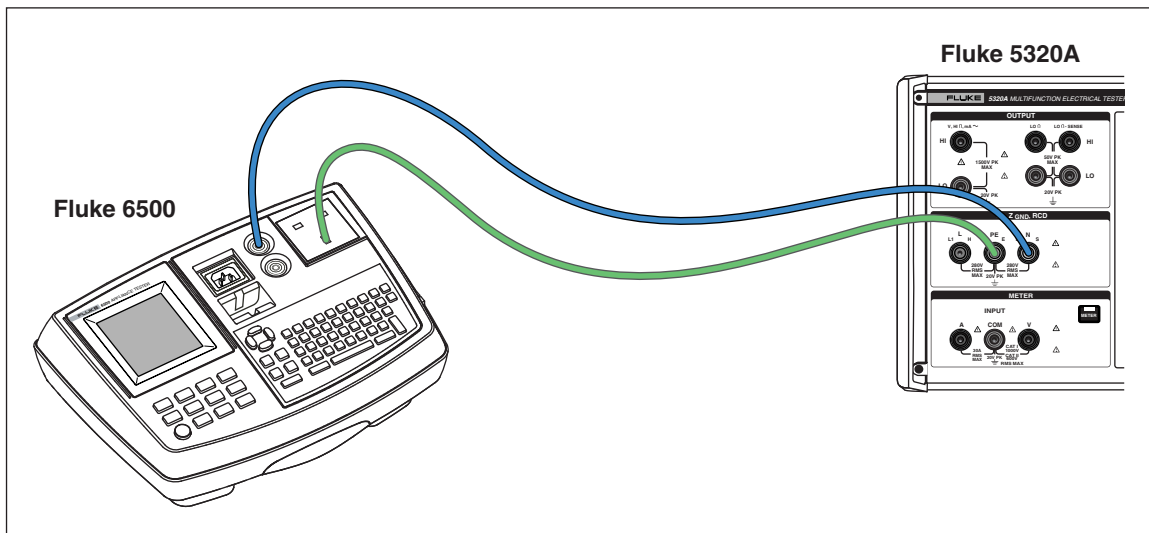
图7-10.使用单独测试导线在 Fluke 6500 上进行接地连接电阻校准
