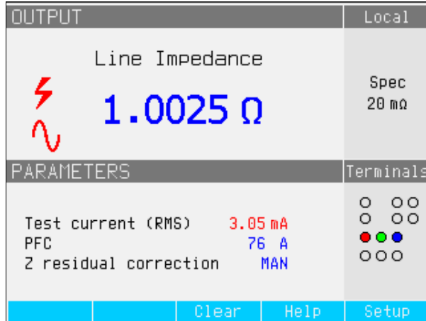
图4-11.电源线阻抗校准显示
