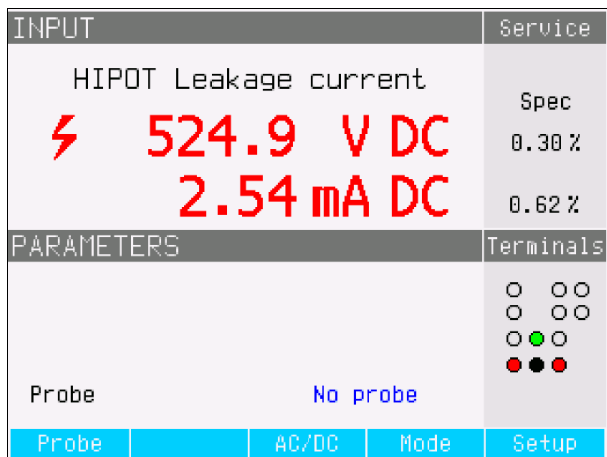
图7-27.泄漏电流校准器显示
