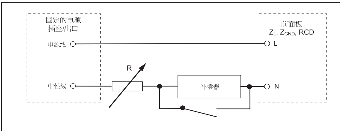
图4-9.简化的电源线阻抗源示意图
