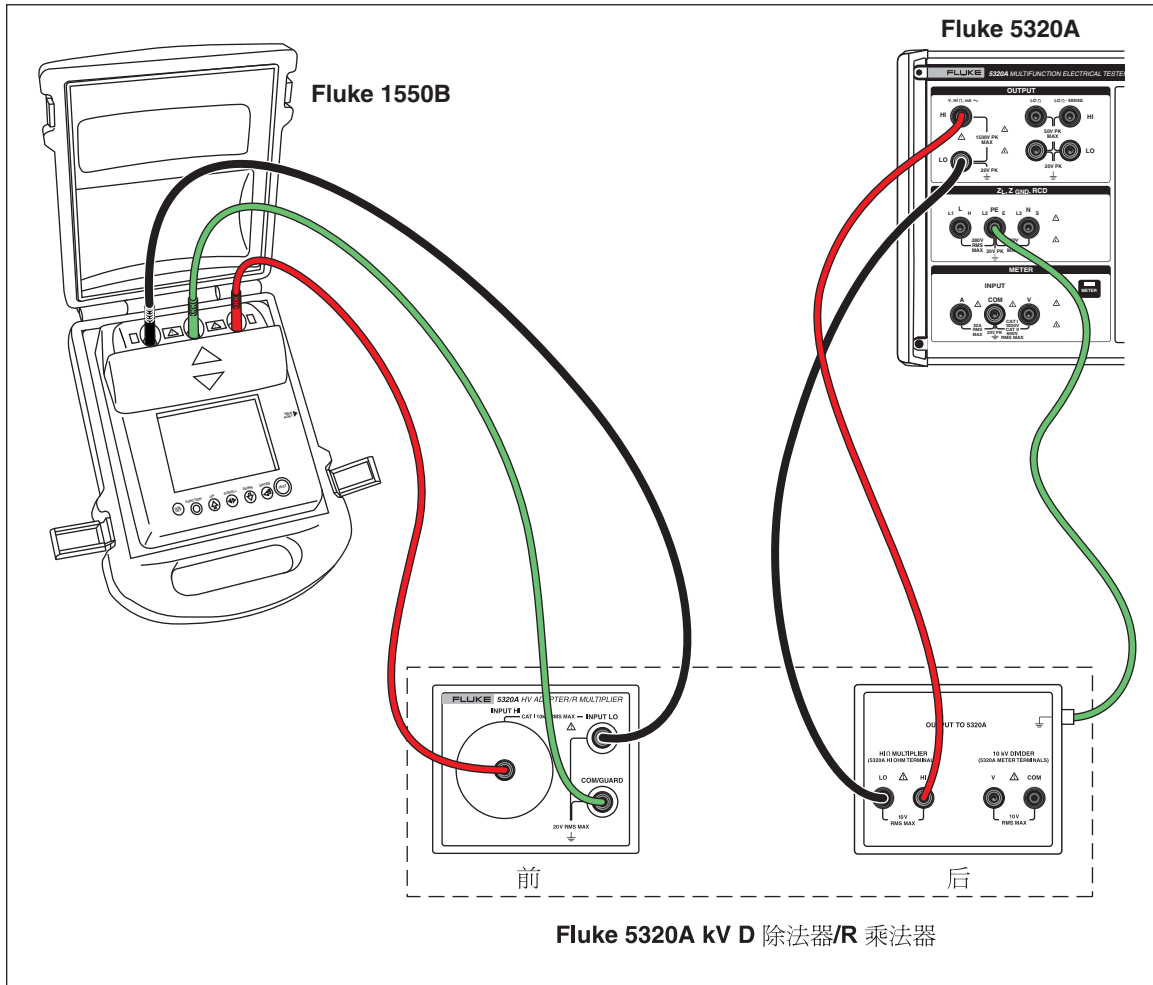
图7-8.当使用电阻乘法器适配器时，到 1550B 的连接
