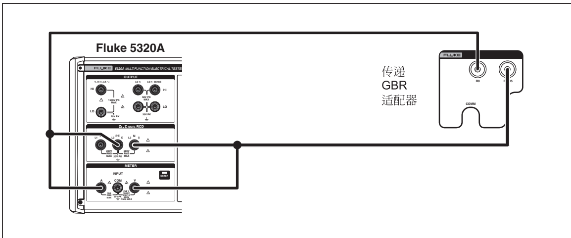
图4-7.有传递负载适配器的接地连接电阻
